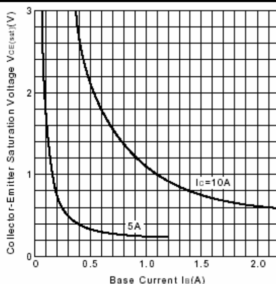
Fig.4 V_{CE(sat)}-I_B
