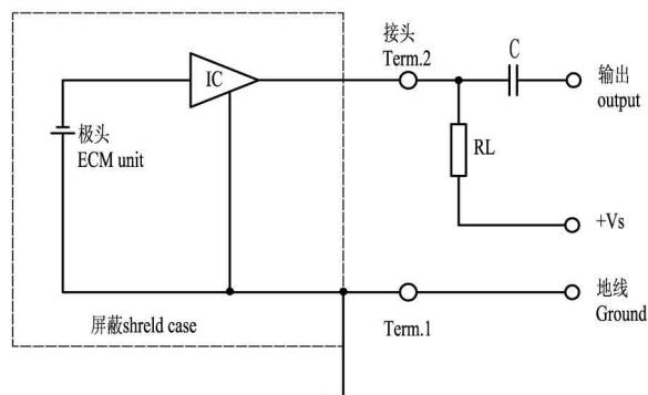
原理图
